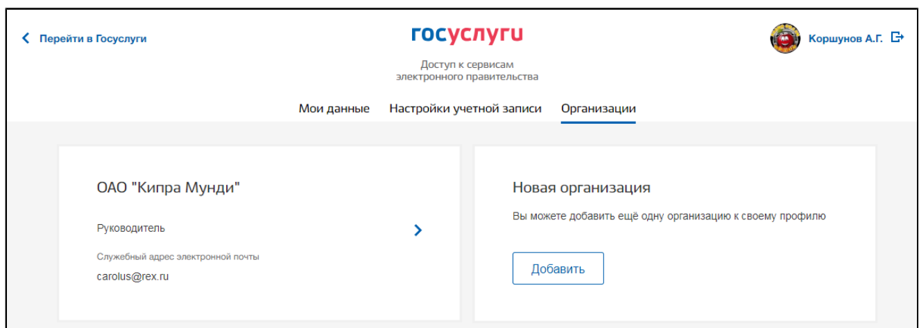
Рис. 46 Вкладка «Организации»
